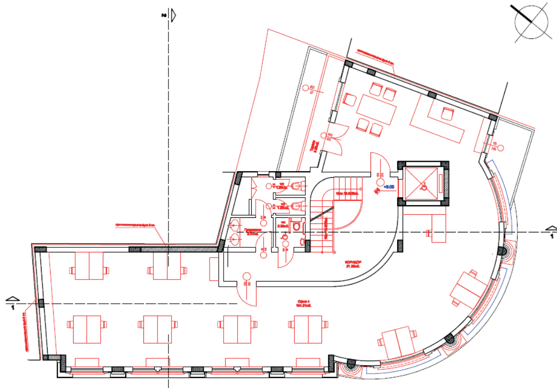
етаж 4, площ 230.30 m 2
