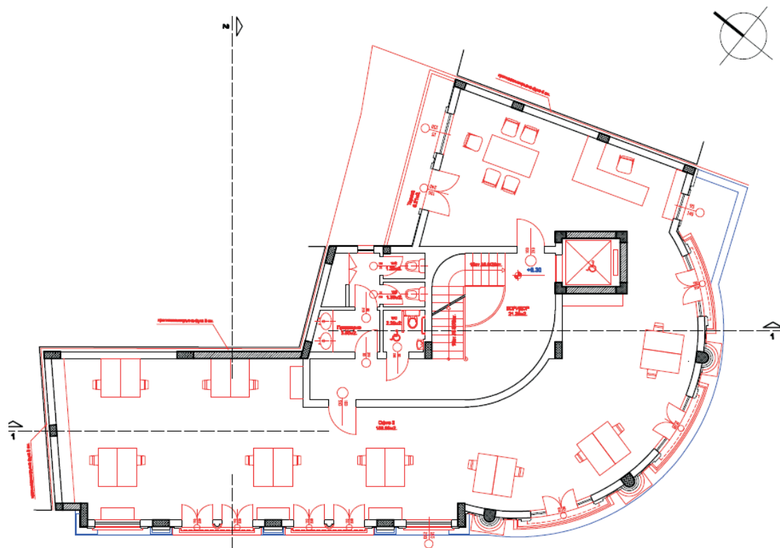
етаж 3, площ 236.37 m 2
